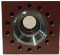
吸入阀箱 Suction Module 单重 Weight: 433 KG · 锻造合金钢
