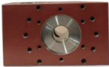
排出阀箱 Discharge Module 单重 Weight: 1,041 KG · 锻造合金钢
